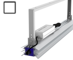
1. Скоба поворотная
